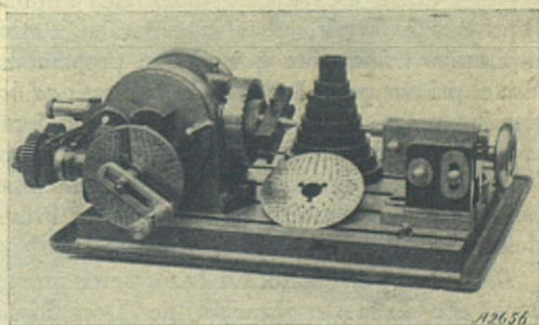
Trabajo de examen. Divisor universal para fresadora universal.
