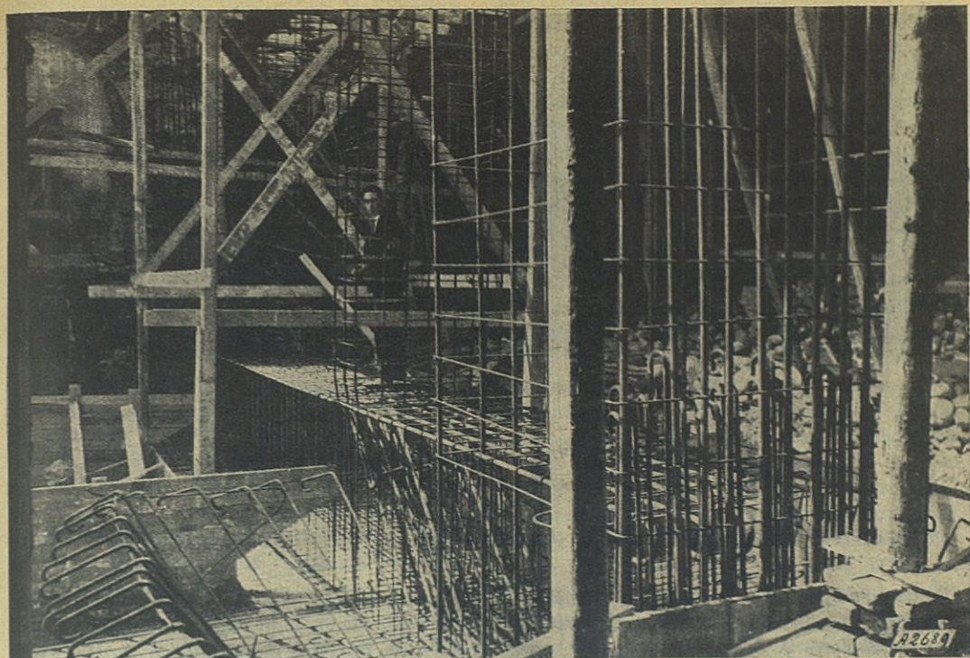
Las obras de la Basílica. - Cómo ha habido que asegurar los cimientos de los pilares que han de llevar la nueva cúpula.
