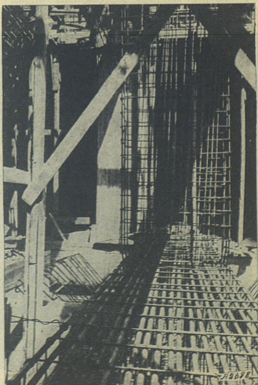
Las obras de la Basílica. - Cómo ha habido que asegurar los cimientos de los pilares que han de llevar la nueva cúpula.
