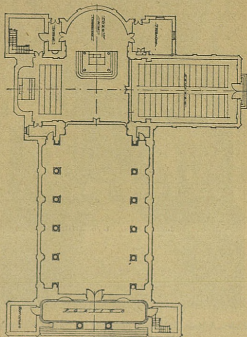
Perú. Plano del Santuario Nacional al Sagrado Corazón.
